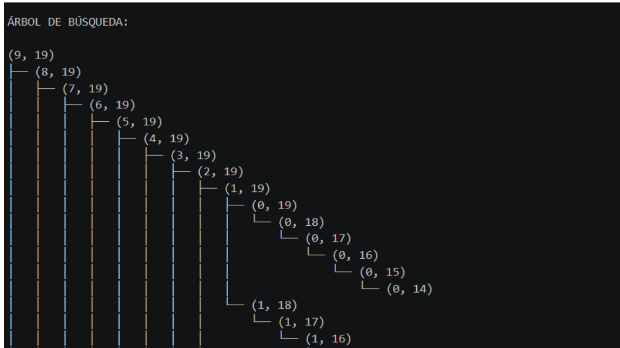
Figura 8: Parte del árbol de búsqueda generados por la búsqueda bidireccional desde el objetivo.
