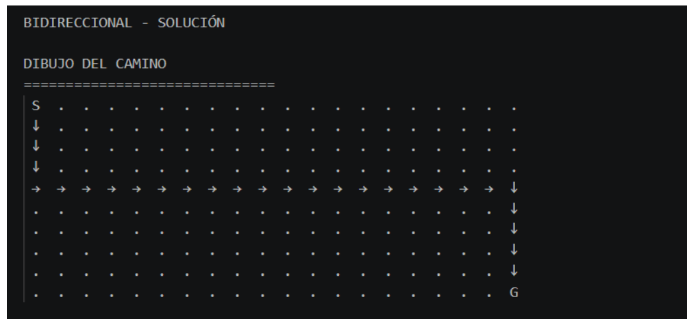
Figura 9: Camino encontrado por la búsqueda bidireccional.
